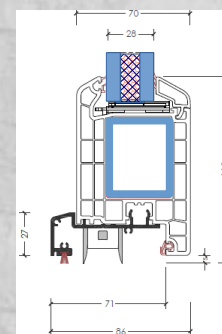
Lama parafreddo
