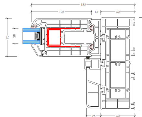
sezione laterale
