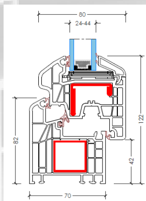
Battente semicomplanare
