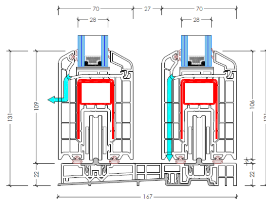
sezione inferiore
