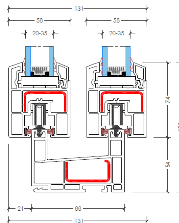
sezione inferiore
