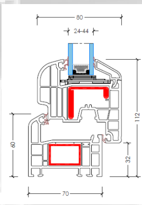
Battente semicomplanare
